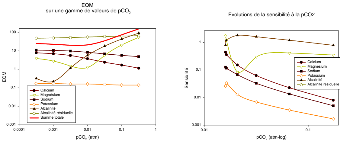
FIG. 7.6: EQM et sensibilité aux valeurs de pCO_2
