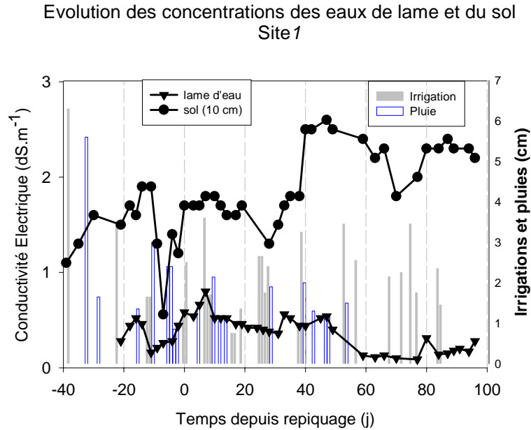
FIG. 9.17: évolution de la concentration des eaux en surface de la parcelle site 1
