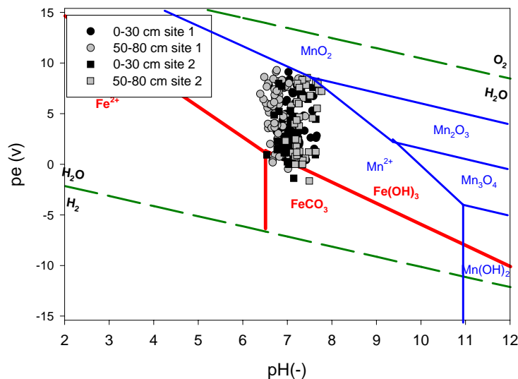
Diagramme de stabilité pH-pe sites 1 et 2, hivernage 1998
