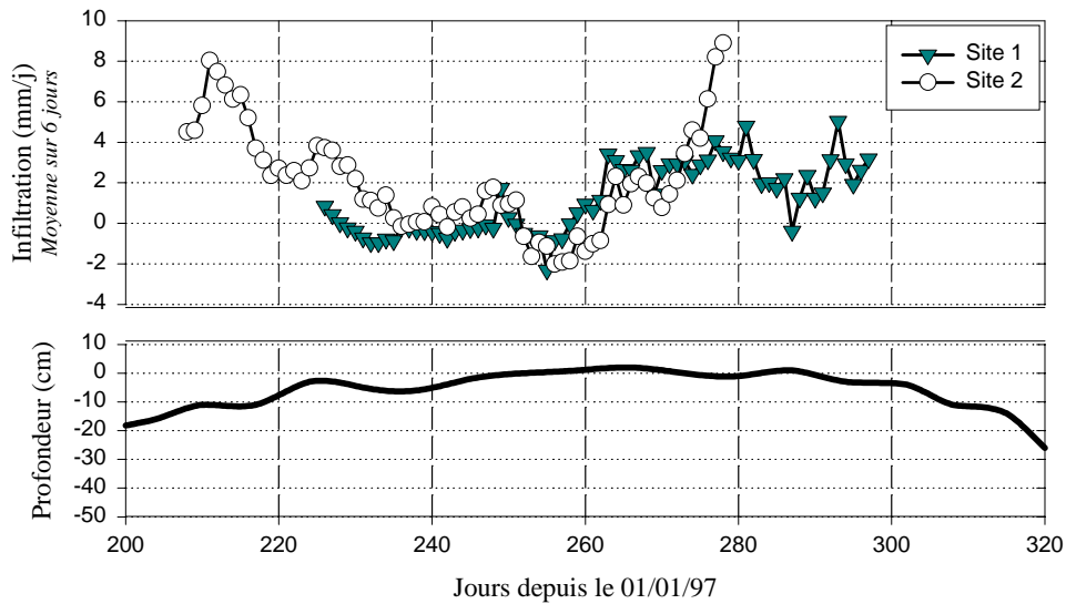
Evolution des vitesses d'infiltration de l'eau Evolution de la profondeur de nappe site 1 et 2, hivernage 1997
