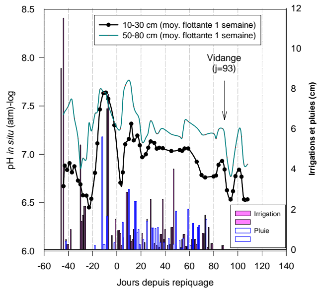
FIG. 9.2: Evolution du pH in situ - sites 1 et 2
