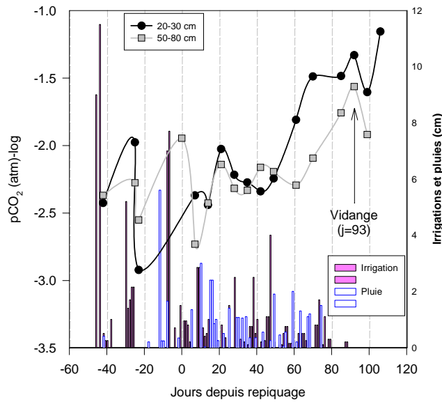
FIG. 9.3: Evolution de la pCO 2 in situ - sites 1 et 2
