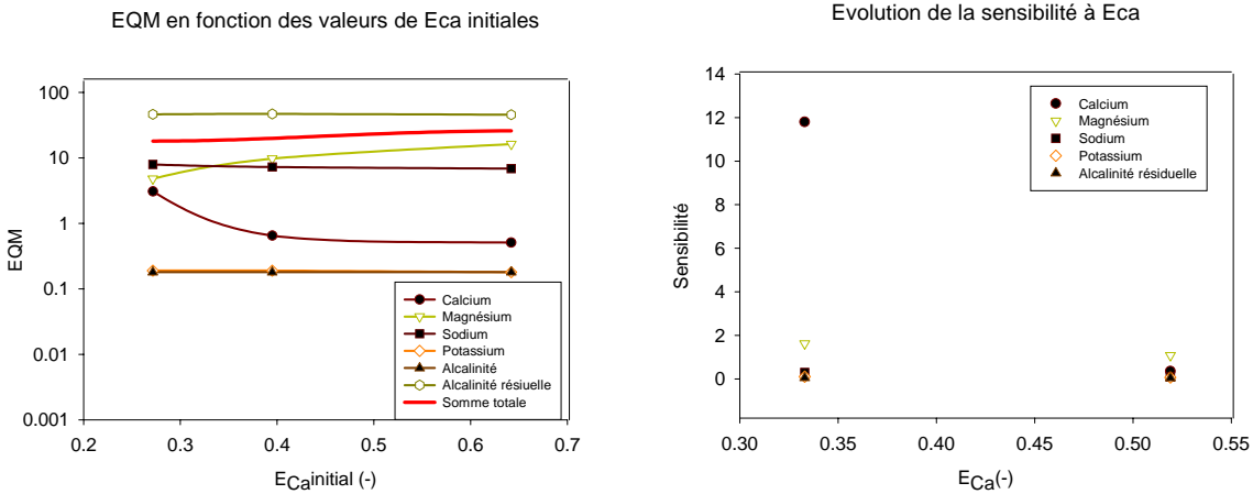
FIG. 7.3: EQM et sensibilité aux valeurs de la fraction de calcium échangeable
