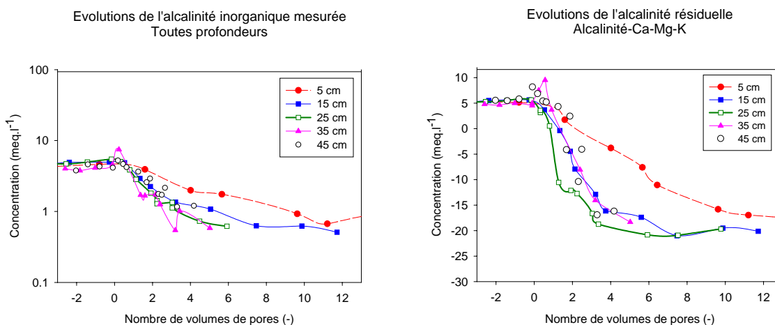
FIG. 6.3: Evolution des concentrations des ions à toutes les profondeurs
